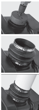
Рис. 9 Подсоединение вертикального подводящего трубопровода 110 мм (DN100)
