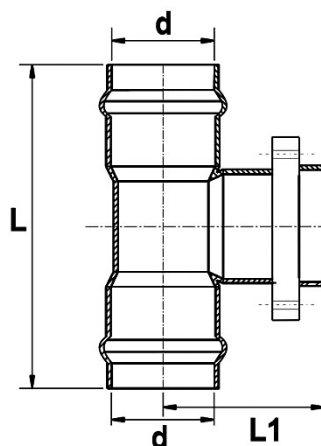
Размеры (мм) и масса (кг) тройников с металлическим фланцем
