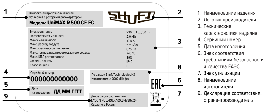
Рис. 4. Пример заводской этикетки
