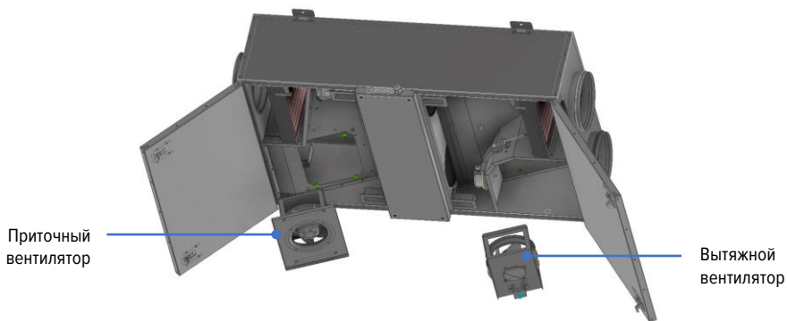
Рис. 29. Обслуживание вентилятора
