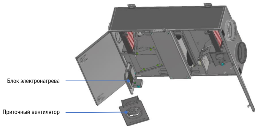
Рис. 30. Обслуживание электронагревателя
