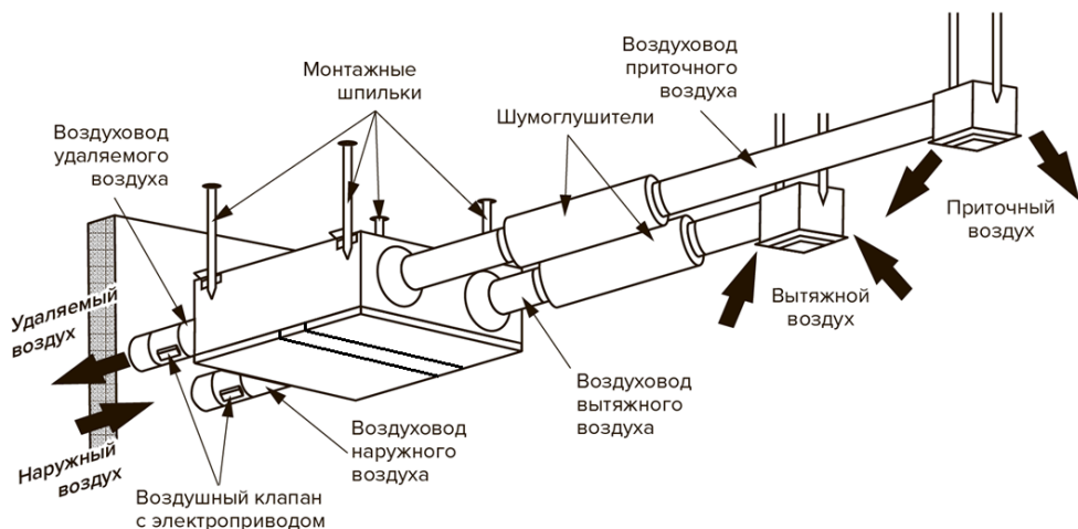
Рис. 11. Монтажная схема
