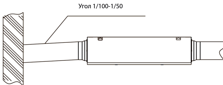
Рис. 10. Уклон наружных воздуховодов
