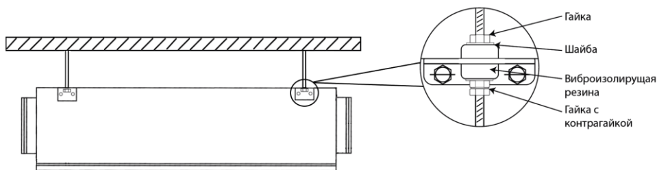
Рис. 5. Монтаж
