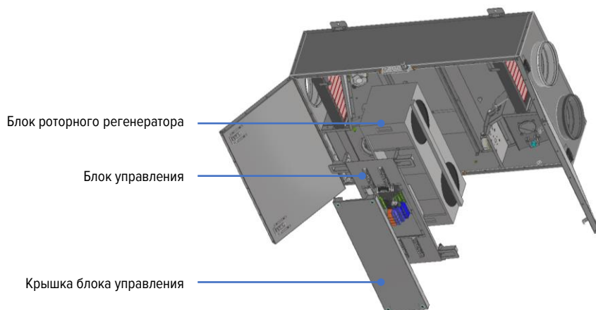
Рис. 28. Обслуживание роторного регенератора
