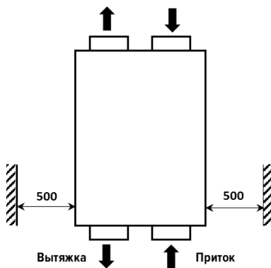
Рис. 7. Сервисное пространство сбоку
