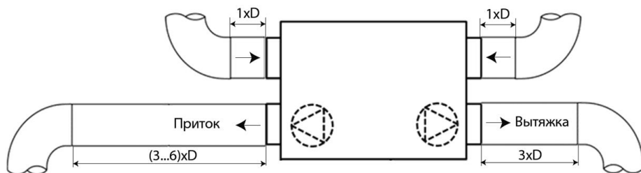
Рис. 8. Рекомендации по длине прямых участков воздуховода
