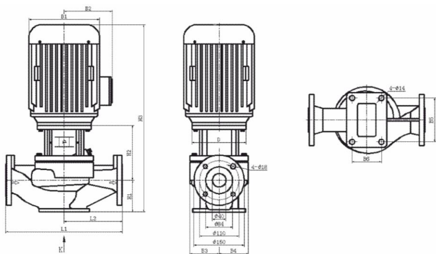
Рис. 20г. Габаритно-присоединительные размеры модели TD(I)40
