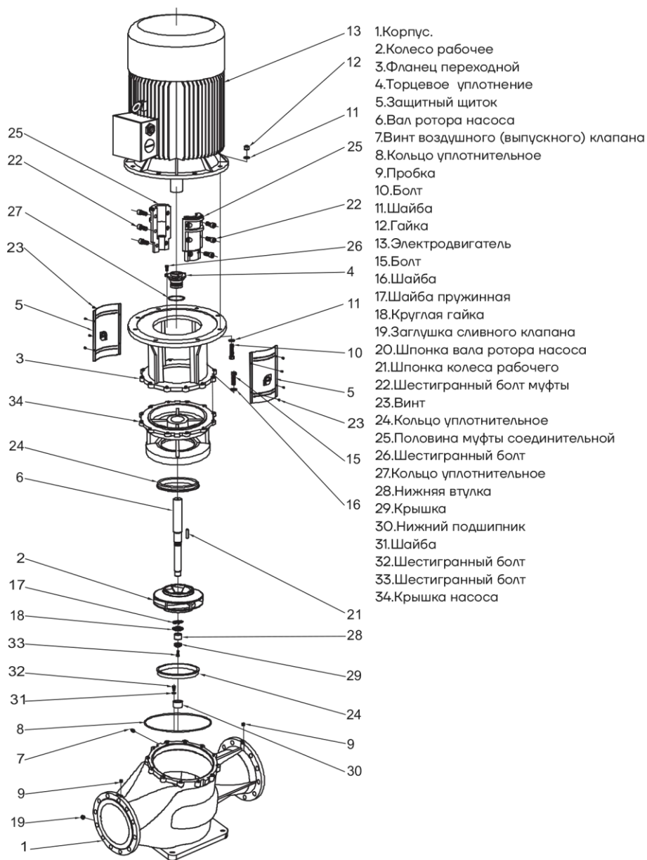
Рис. 18-С TD300-TD350
