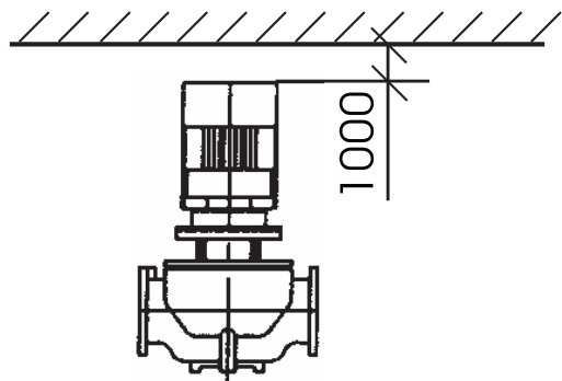
Рис. 10 Электродвигатель > 5 кВт
