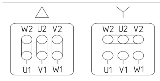
Рис. 15 Схема клеммных соединений
