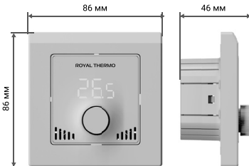
Рис. 1. Габариты терморегулятора
