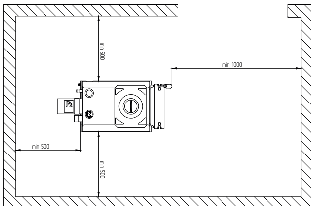
Рис.2. Схема установки аппарата «Profi-X».
