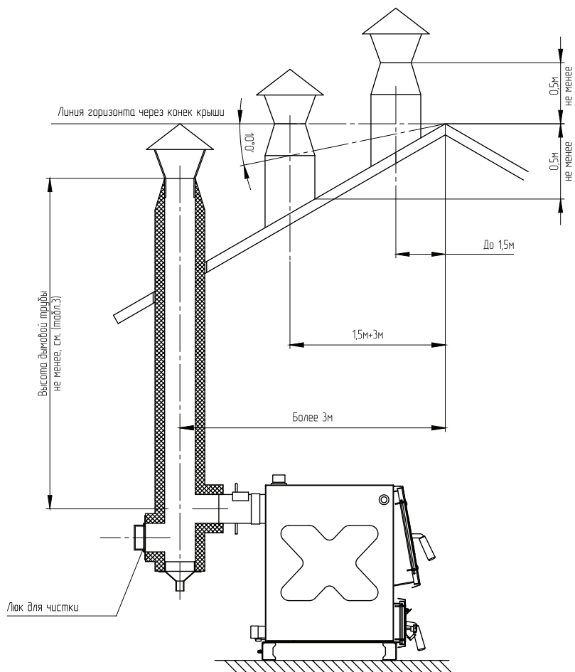
Рис.3. Варианты установки дымоходной трубы.
