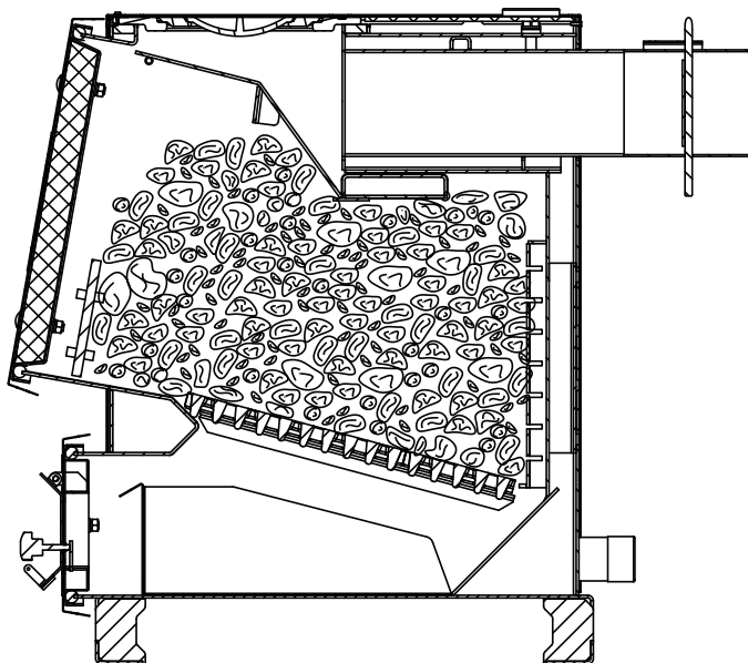
Рис.6. Схема загрузки аппарата «Profi-X».
