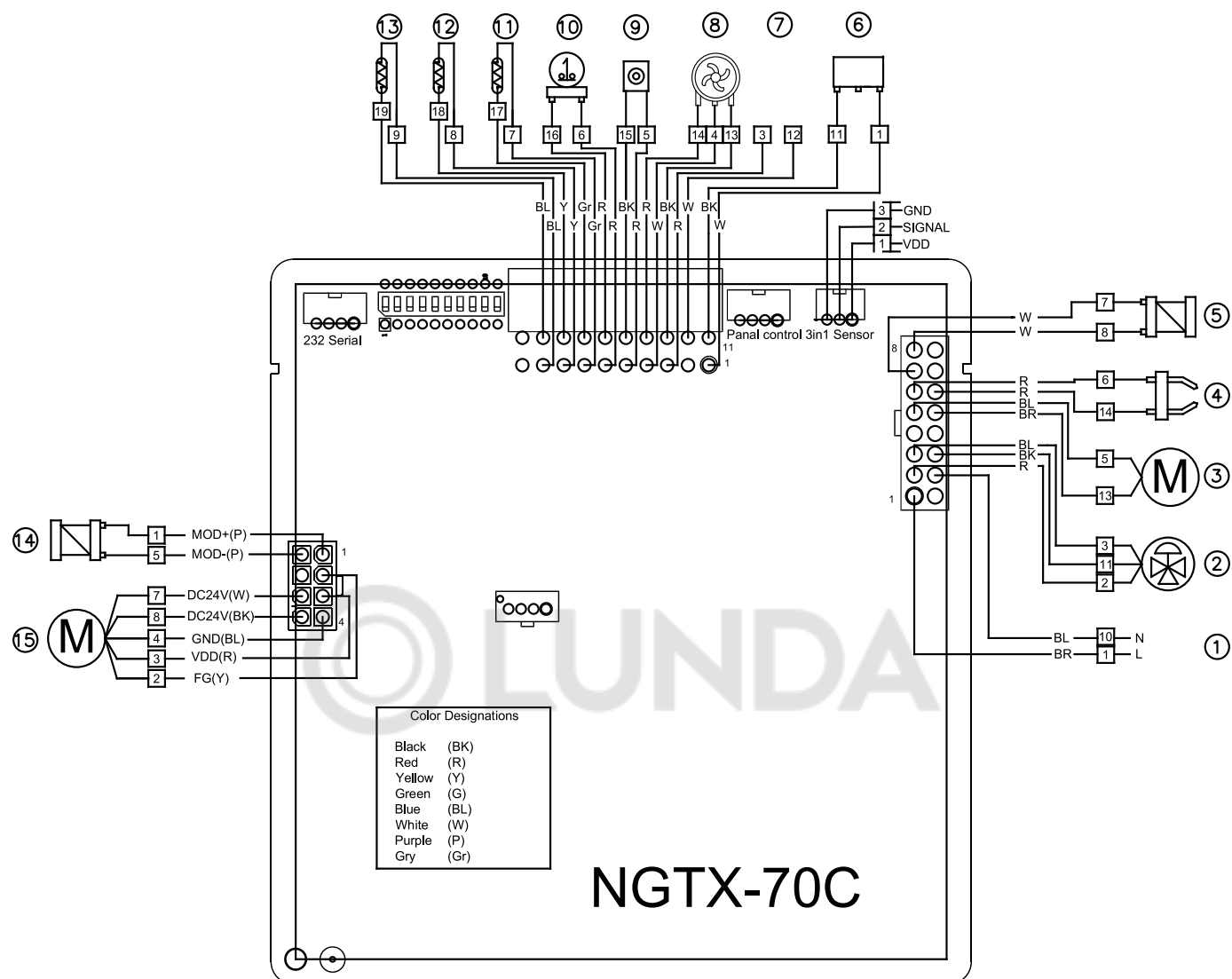
Рисунок 14. Схема электрическая.
