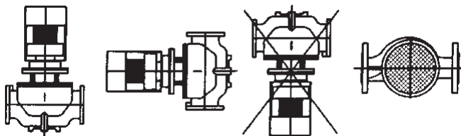
Рис. 7 Варианты установки \leq 2,2 кВт
