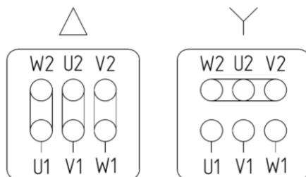
Рис. 15 Схема клеммных соединений
