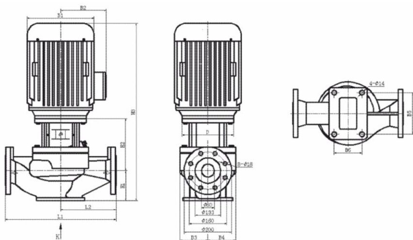
Рис. 20з. Габаритно-присоединительные размеры модели TD(I)80
