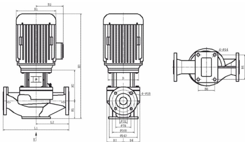
Рис. 20в. Габаритно-присоединительные размеры модели TD32-12,5(I)/2, TD32-15(I)/2
