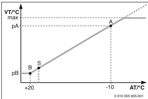
Рис. 2 Отопительная кривая
