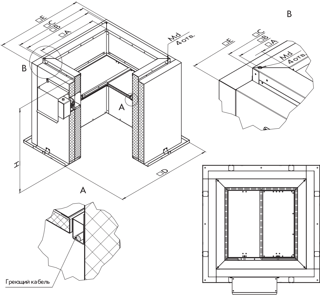
СТМ 204 ДУ УХЛ / 214 ДУ УХЛ
