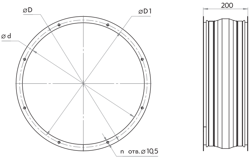
Гибкая вставка «В» типа «фланец-фланец»
