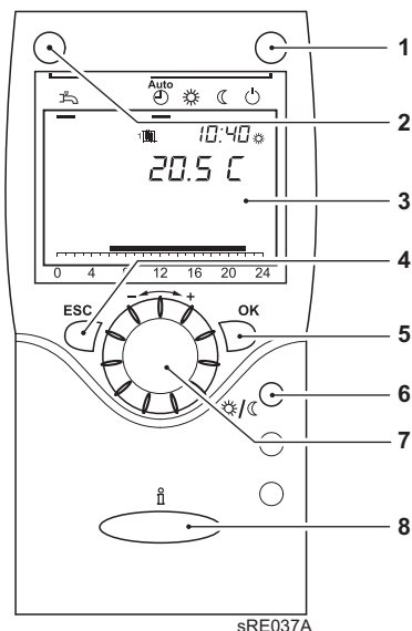
Рис.2 Интерфейс комнатного устройства RGT
