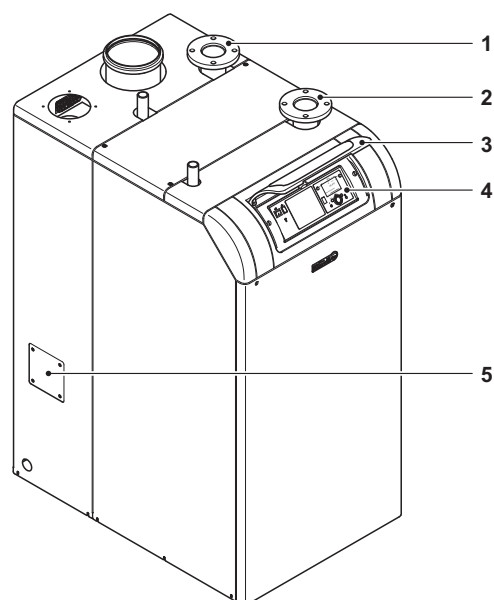
Рис.1 Обзор Power HT 1.130 - 1.320
