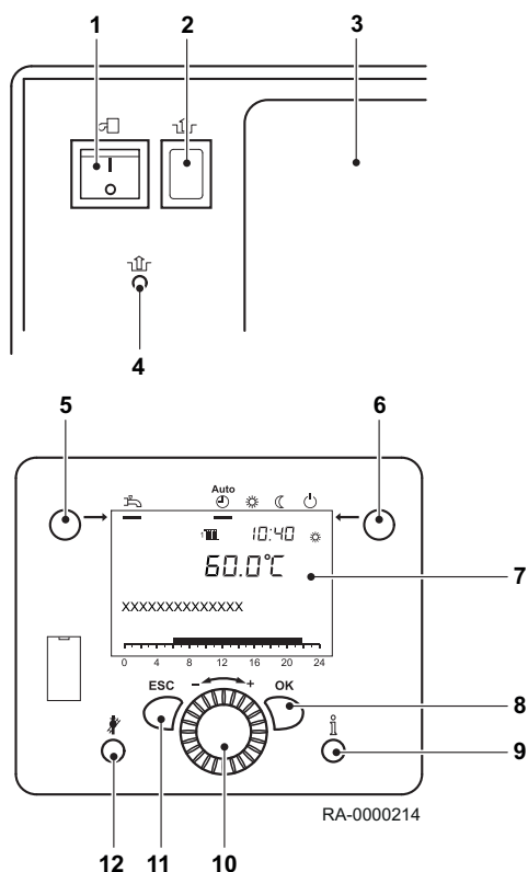
Рис.3 Функциональные элементы
