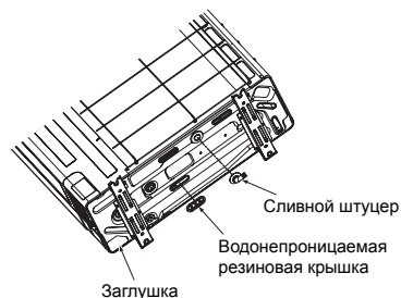
Сливной штуцер
