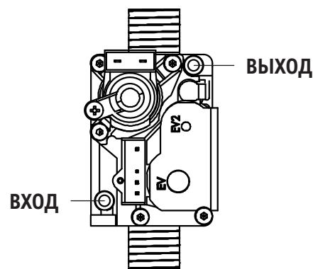
Штуцеры замера давления газа
