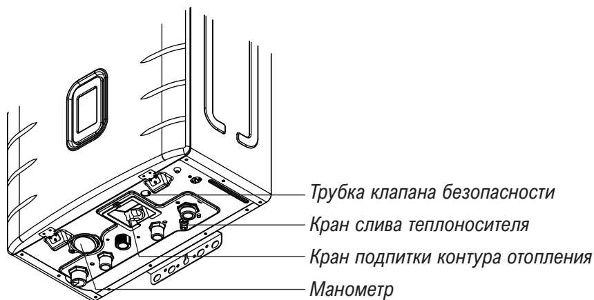
Рисунок 5. Схема нижней панели котла.
