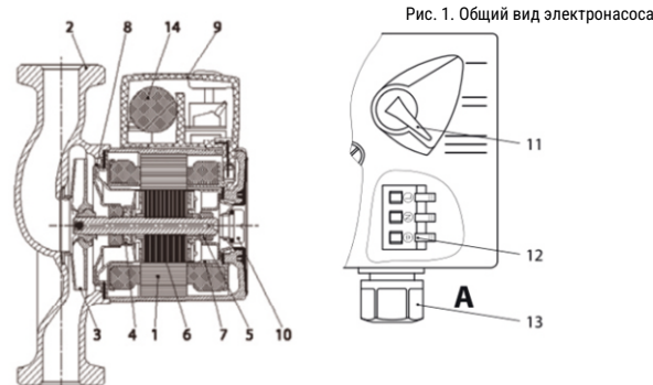
Рис. 1. Общий вид электронасоса
