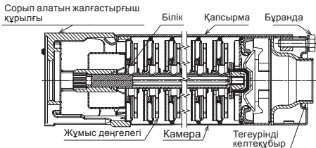
2-сур. Электр қозғалтқышсыз сыртқа тебу орындалымындағы SQF сорғыларының түрі.
