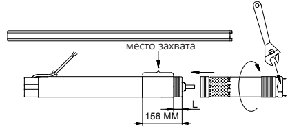
Рис. 13 Затяжка насоса
