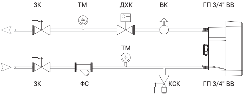
Рекомендованная схема подключения тепловентилятора к системе отопления с использованием двухходового клапана
