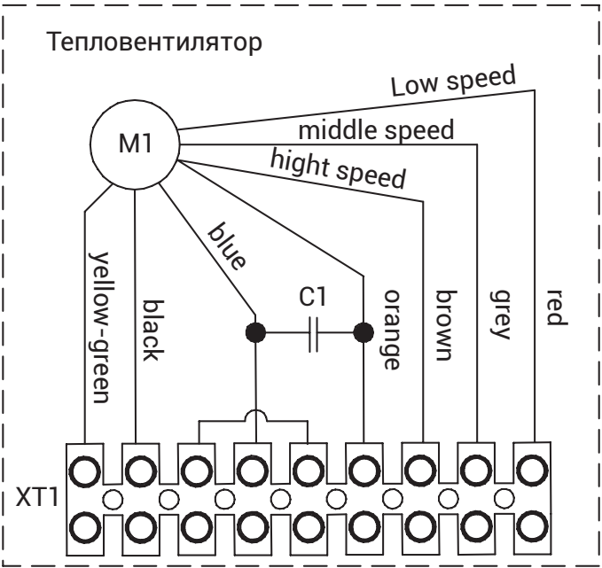
Внутренняя схема клеммной коробки тепловентилятора.
