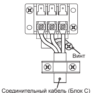
* Пример подключения (RAS-3M26G3AVG-E)
