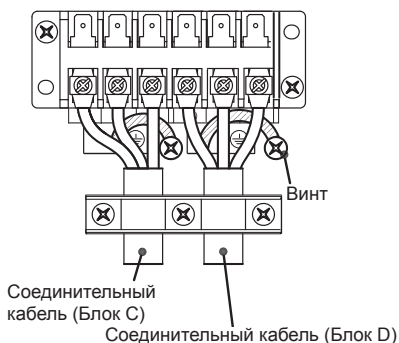
* Пример подключения (RAS-4M27G3AVG-E)
