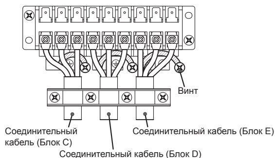
* Пример подключения (RAS-5M34G3AVG-E)
