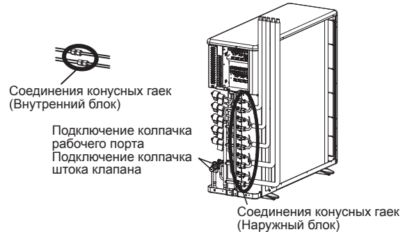
* Пример контрольной точки (RAS-5M34G3AVG-E)
