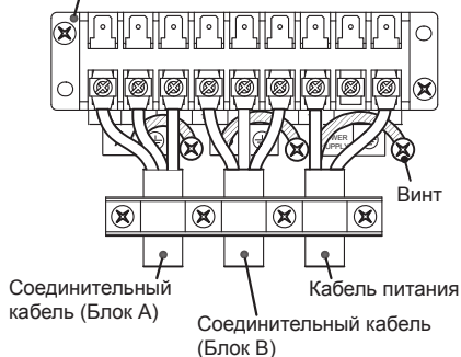
Клемная колодка (Соединительный кабель)
