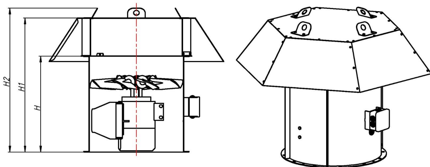
Рисунок 1. Габаритные и присоединительные размеры вентилятора
