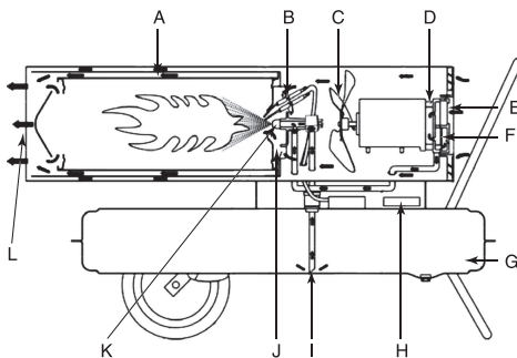
Рис. 9. Устройство защиты.
