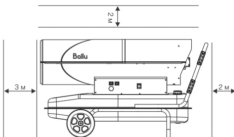
Рис. 6. Безопасные дистанции.
