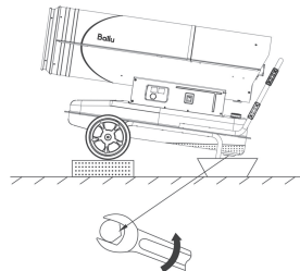
Рис. 10. Опорожнение топливного бака.
