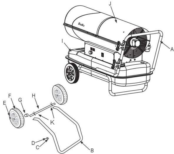
Рис. 4. Установка колес и каркаса.
