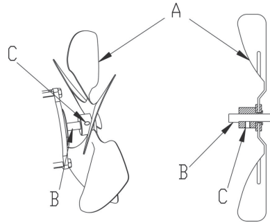
Рис. 13. Крепление крыльчатки.
