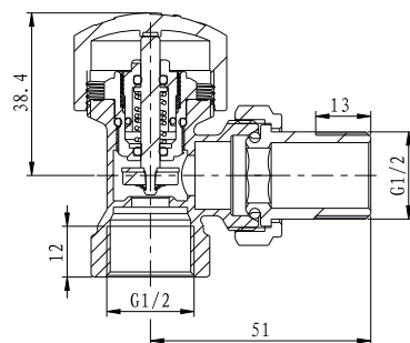
Угловой термостатический клапан
