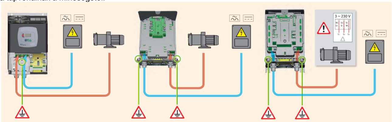
4.ábra: Elektromos bekötések
