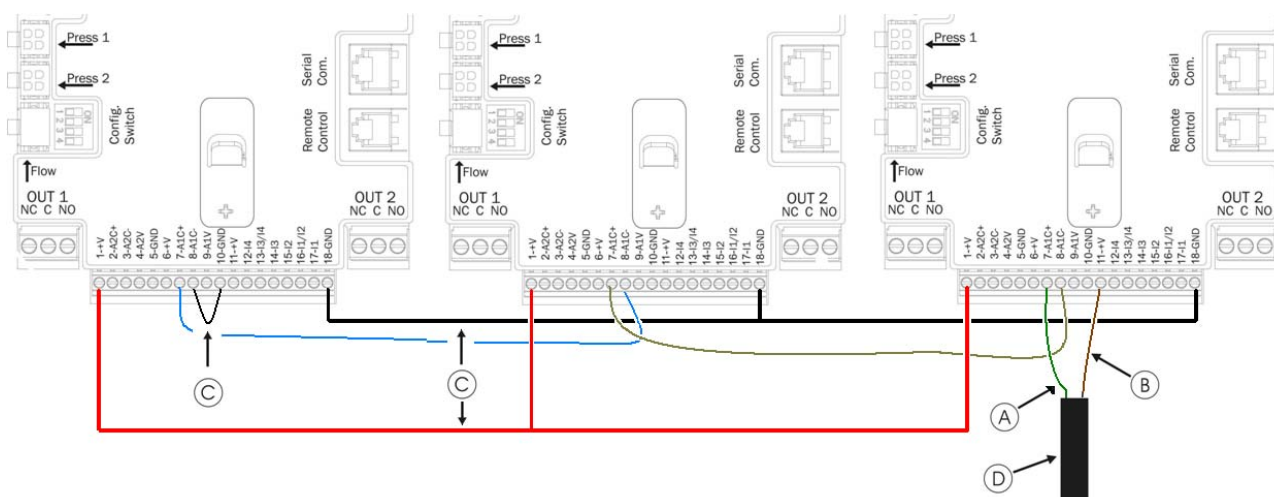
Фигура 9: Свързване на датчик за налягане по ток 4 - 20 mA за мултиинвертор
