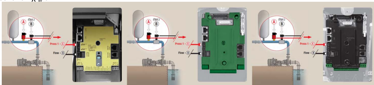
Σχήμα 7: Συνδέσεις αισθητήρων
