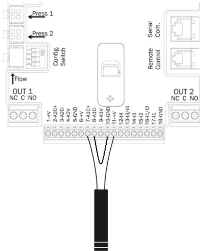
Фигура 8: Свързване на датчик за налягане по ток 4 - 20 mA
