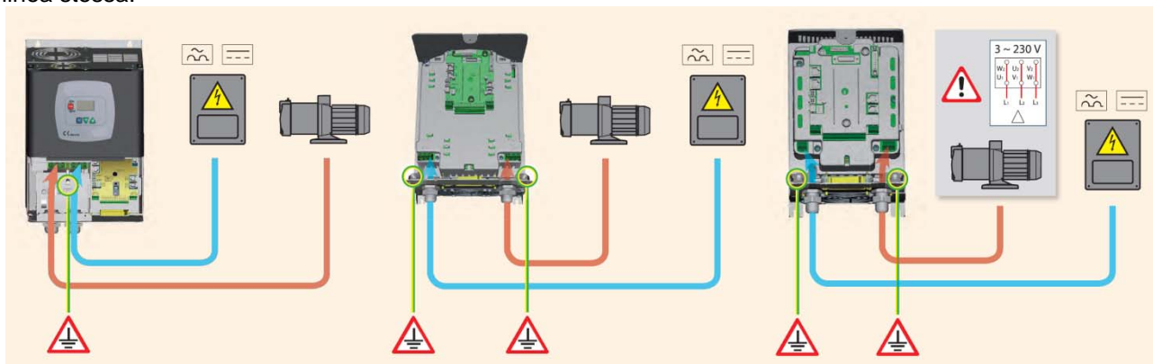
Figura 4: Connessioni elettriche
