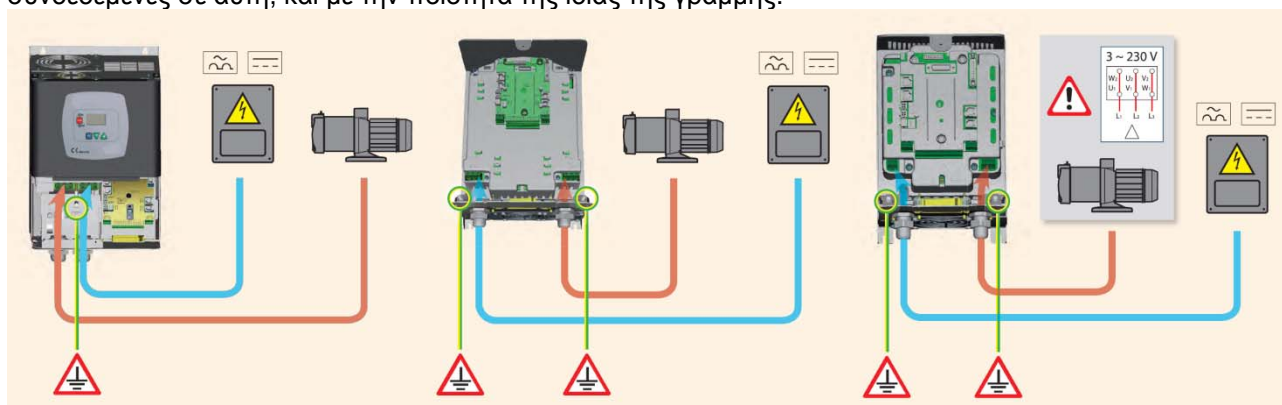
Σχήμα 4: Ηλεκτρολογικές συνδέσεις
