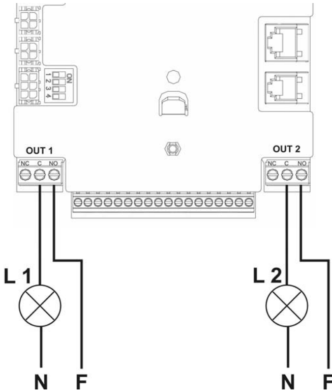
Şekil 10: bağlantıları örneği
