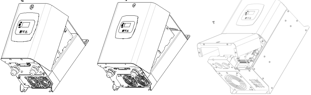
Şekil 3: Bağlantılara erişim için kapağın sökülmesi
