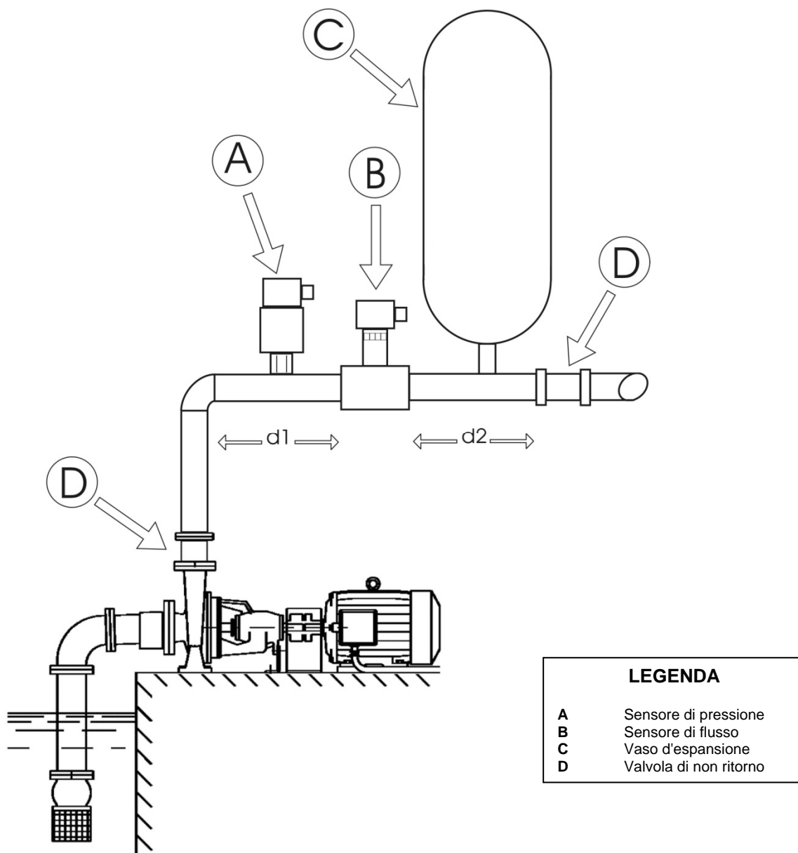
Figura 6: Installazione Idraulica
