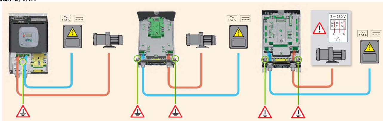
Rys. 4: Podłączenia elektryczne
