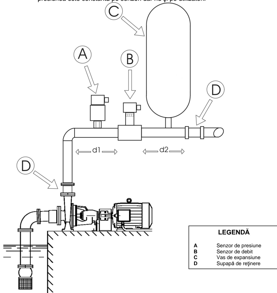
Figura 6: Instalația hidraulică
