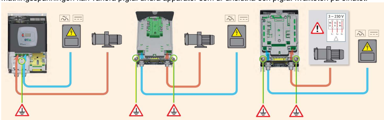
Fig. 4: Elanslutning
