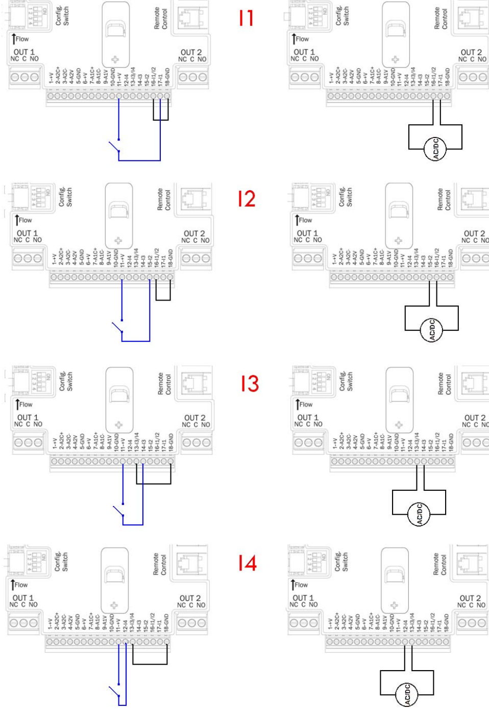
Şekil 11: bağlantıları örneği
