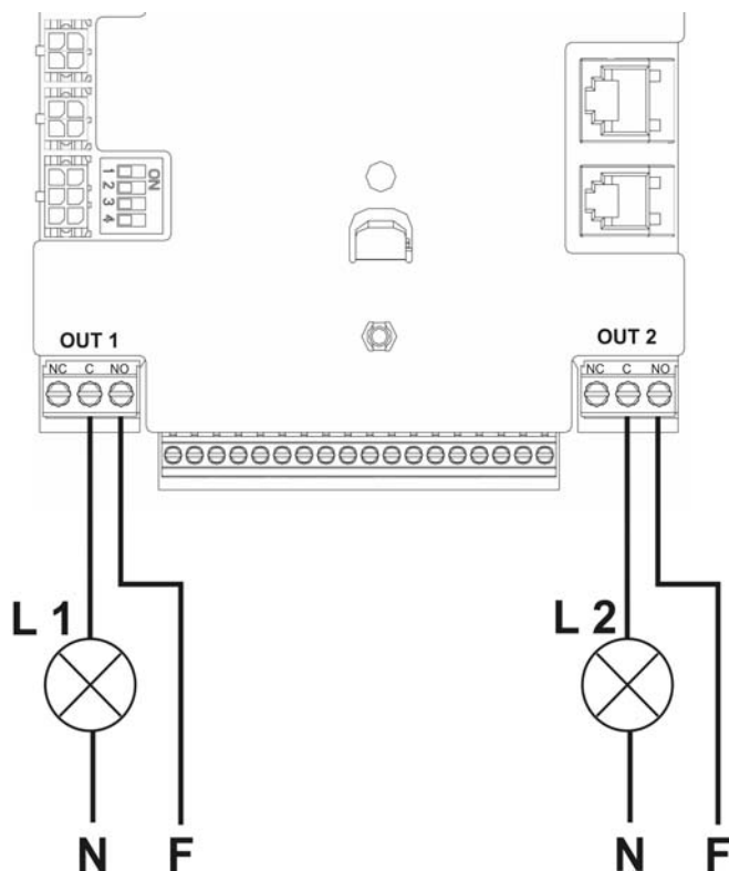
Σχήμα 10: Παράδειγμα σύνδεσης των εξόδων
