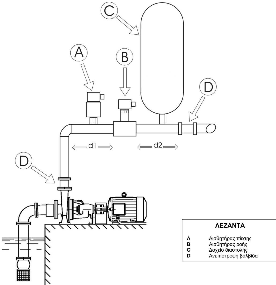
Σχήμα 6: Υδραυλική εγκατάσταση
