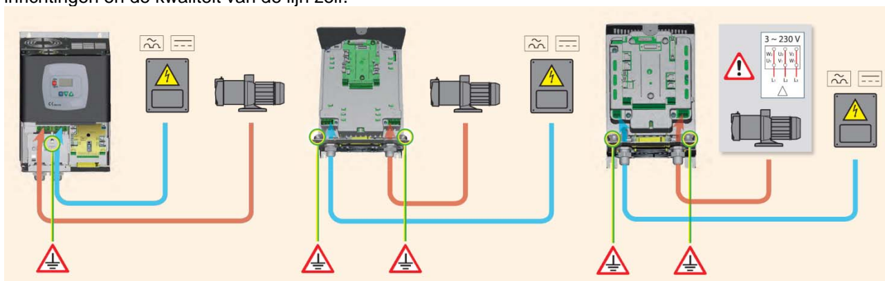
Afbeelding 4: Elektrische aansluitingen
