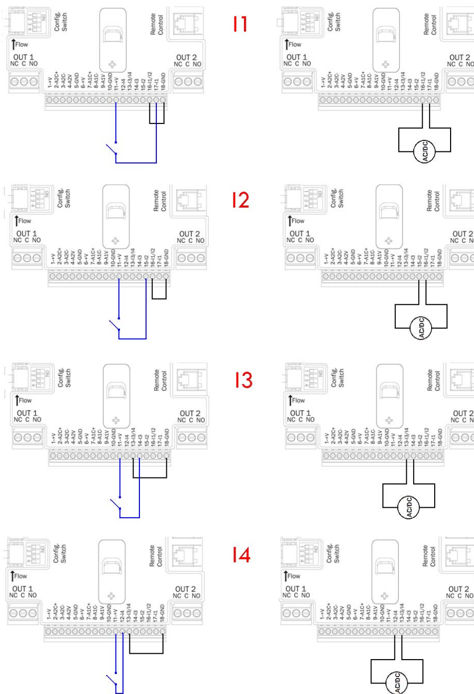
Fig. 11: Exempel på anslutning av ingångar
