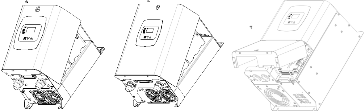
Fig. 3: Demontering av locket för åtkomst till anslutningarna
