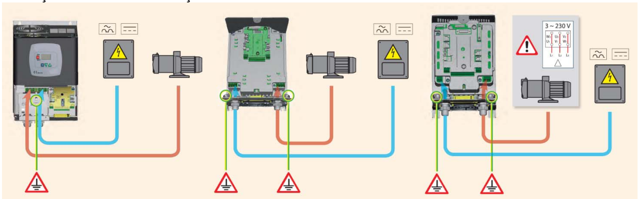
Figura 4: Conectări electrice
