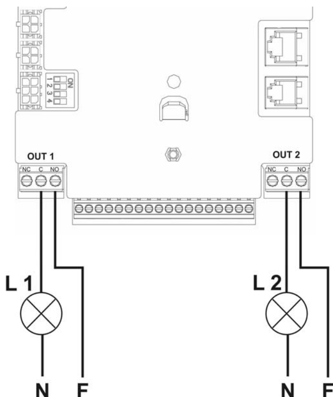
Abbildung 10: Anschlussbeispiel der Ausgänge
