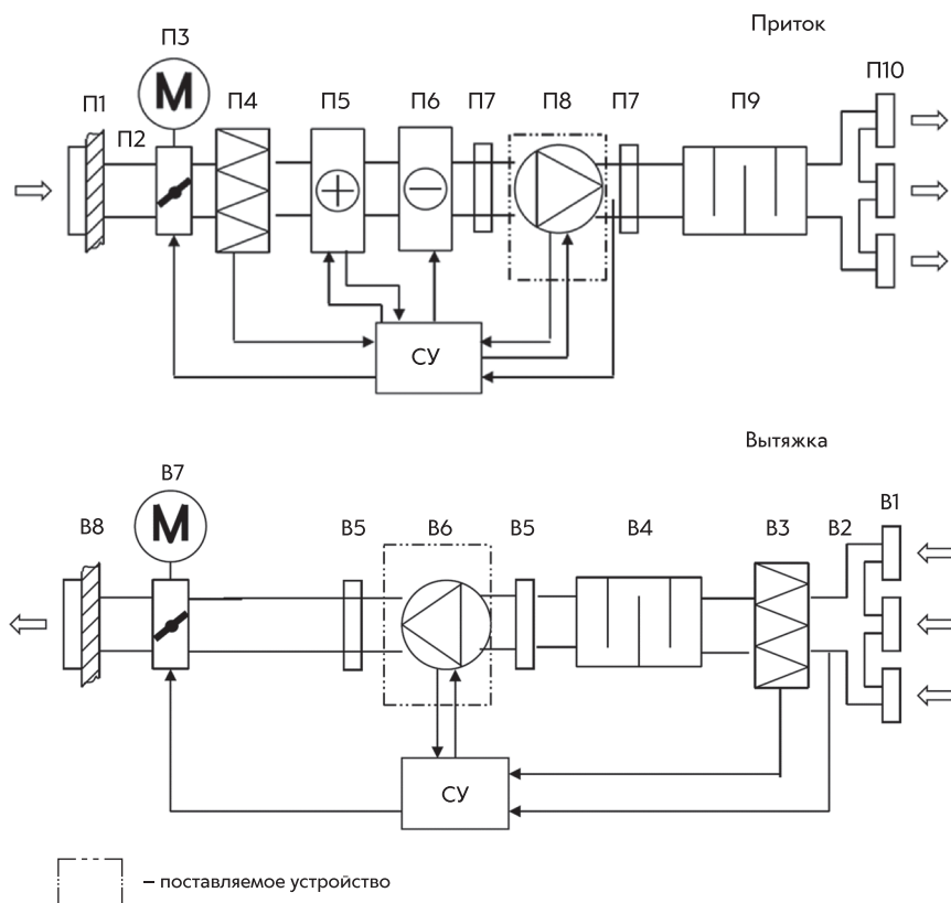
Рис. 1. Структура и состав системы вентиляции.
