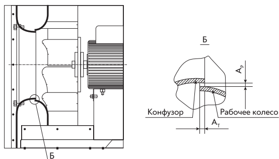
Рис. 3. Зазоры между конфузором и рабочим колесом
