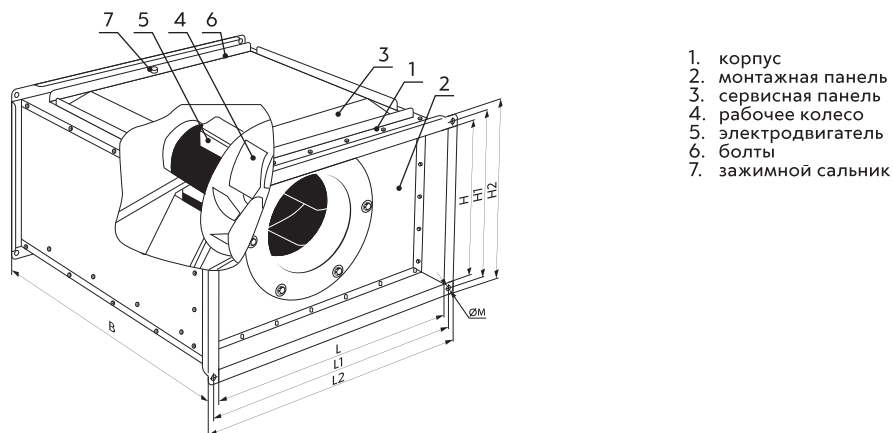
Рис. 2. Состав и габаритные размеры вентилятора.
