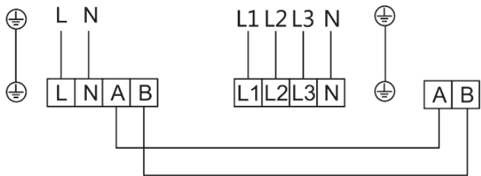
Рис. 63. 48K, 60K (3-фазные блоки)
