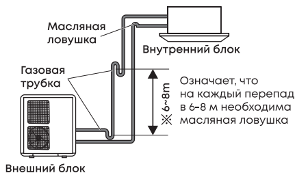
Рис. 58. Наружный блок ниже внутреннего
