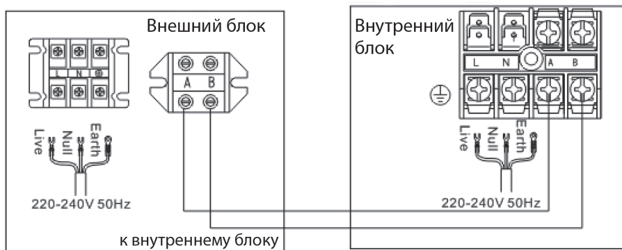
Рис. 62. 12K,18K,24K,36K (1-фазные блоки)
