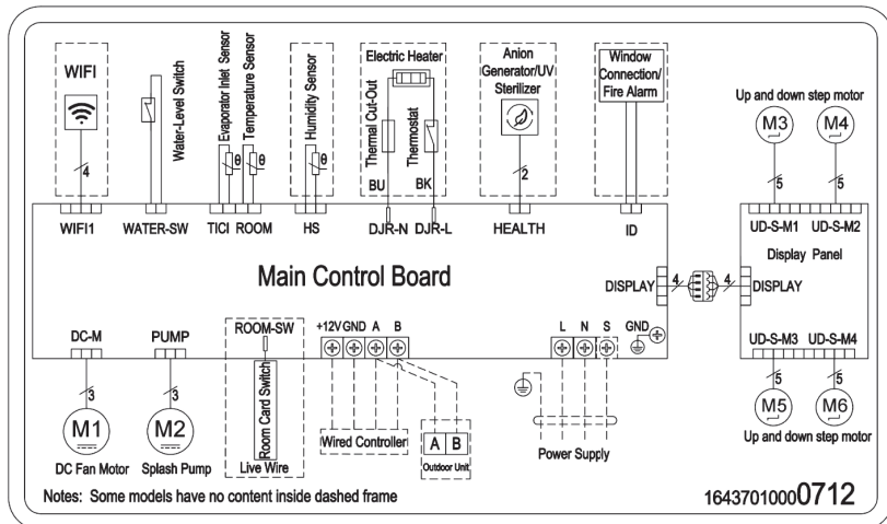
Рис. 65. Кассетные 24К, 36К, 48К, 60К
