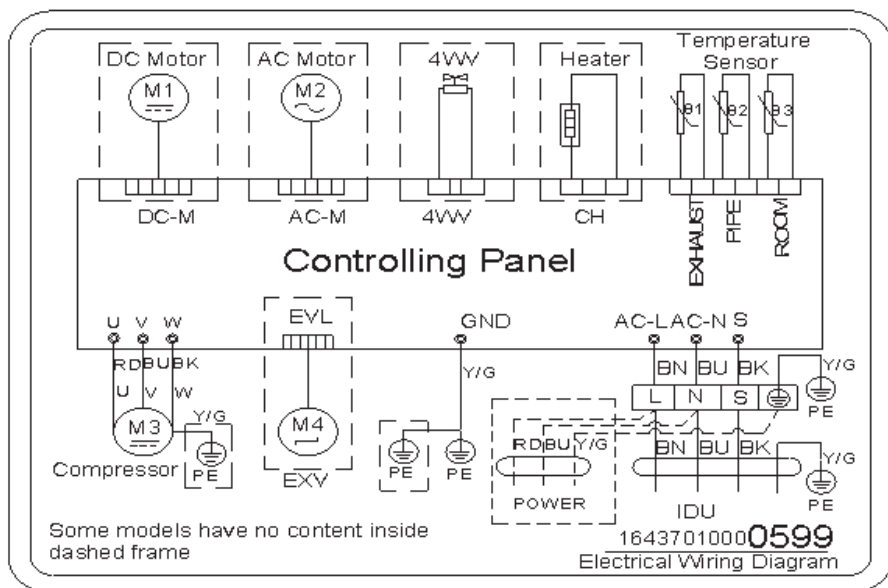
Рис. 67. 18K, 24K, 36K
