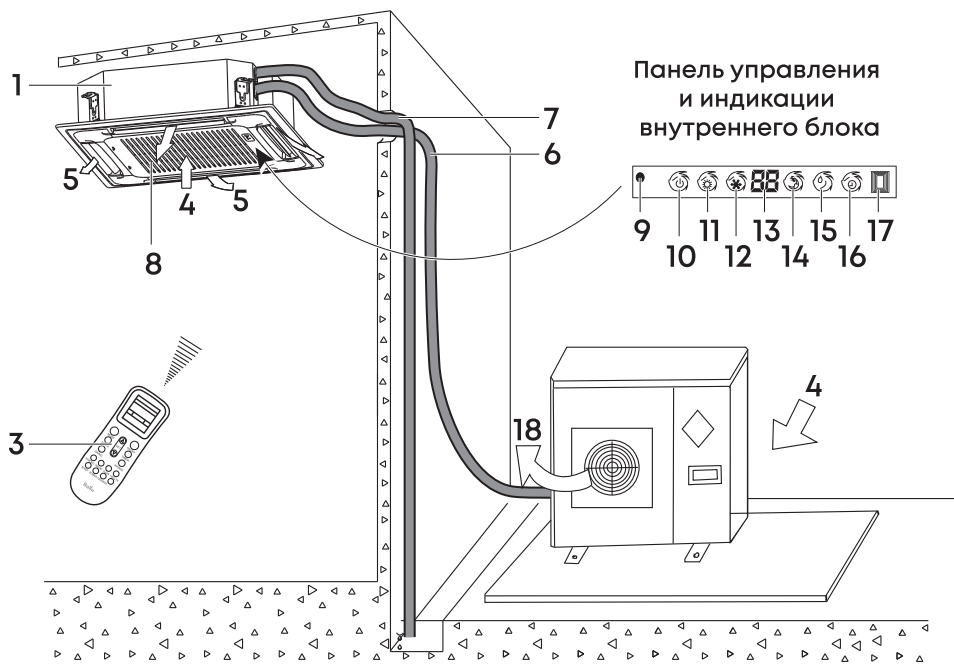
Рис. 1. Устройство кондиционера.*
