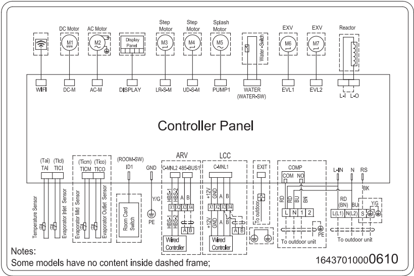
Рис. 64. Кассетные 12K, 18K
