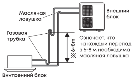
Рис. 59. Наружный блок выше внутреннего
