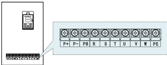
Рисунок 3-9. Схема силовых клемм ПЧ мощностью 11-18,5 кВт.
