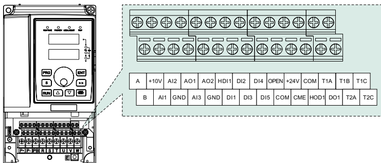
Рисунок 3-17. Клеммы управления.
