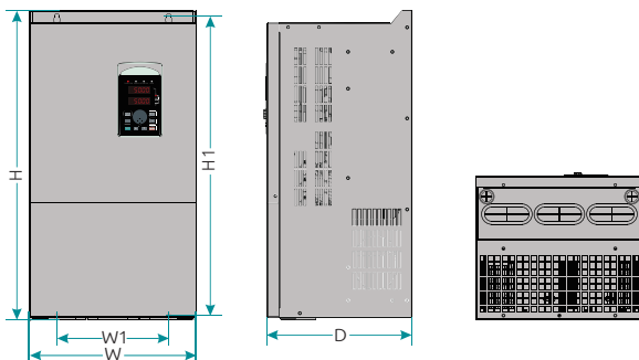
Рисунок 2-8. Установочные размеры ПЧ мощностью до 55 - 110 кВт
