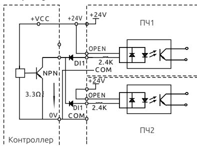
Рисунок 3-20. Параллельное подключение дискретных входов разных ПЧ.
