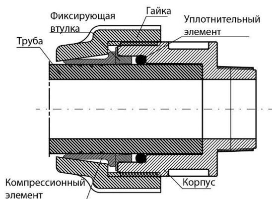
Рисунок 1. Конструкция компрессионной части фитинга.
