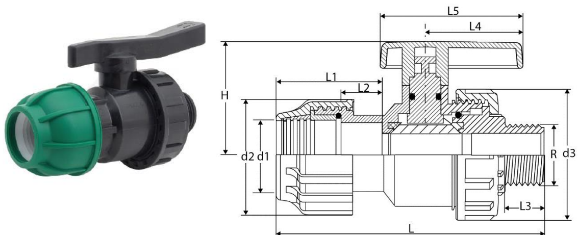
Рисунок 21. Кран шаровой разъемный с наружной резьбой PN 10
