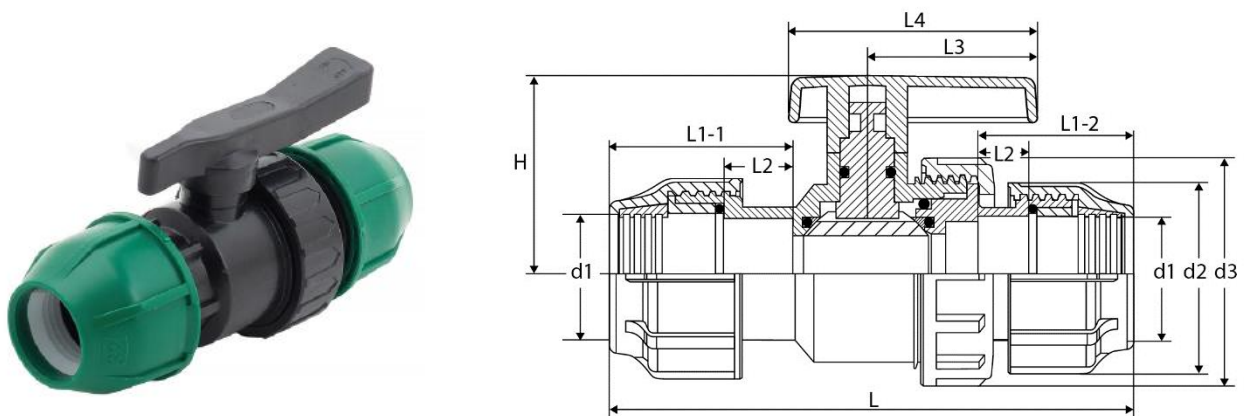
Рисунок 22. Кран шаровой разъемный PN 10
