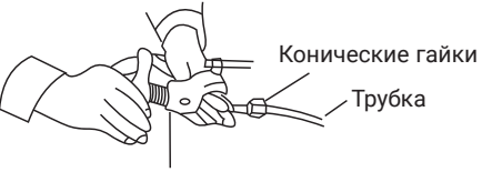
Развальцовочный инструмент
