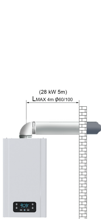
Горизонтальная система дымоудаления (L макс. расстояние с одним коленом: 4 м, Ø60/100) (L макс. расстояние с одним коленом: 6 м, Ø80/125)
