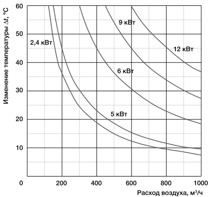
Подбор электронагревателя
