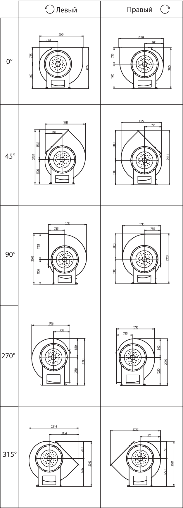
RAD 11,2
