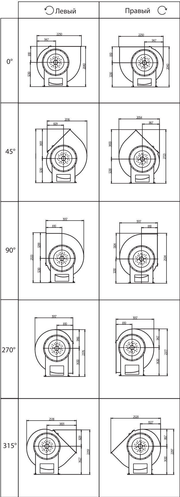
RAD 12,5
