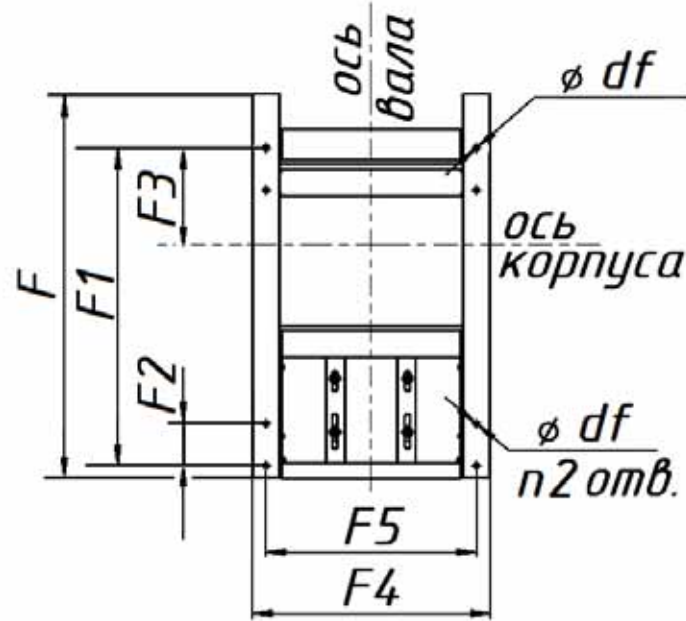
Основание монтажной рамы вид В
