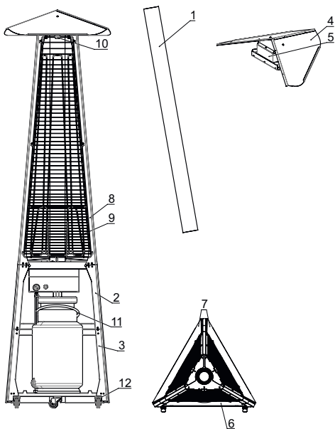
Рис. 2 - Устройство модели
