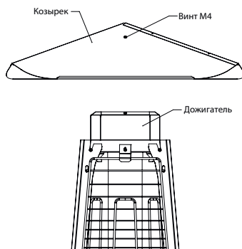
Рис.12 - Установка козырька
