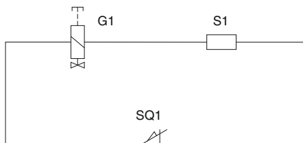
Рис.20 - Схема электрическая принципиальная
