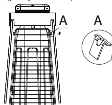
Рис.11б - Установка фиксатора решетки
