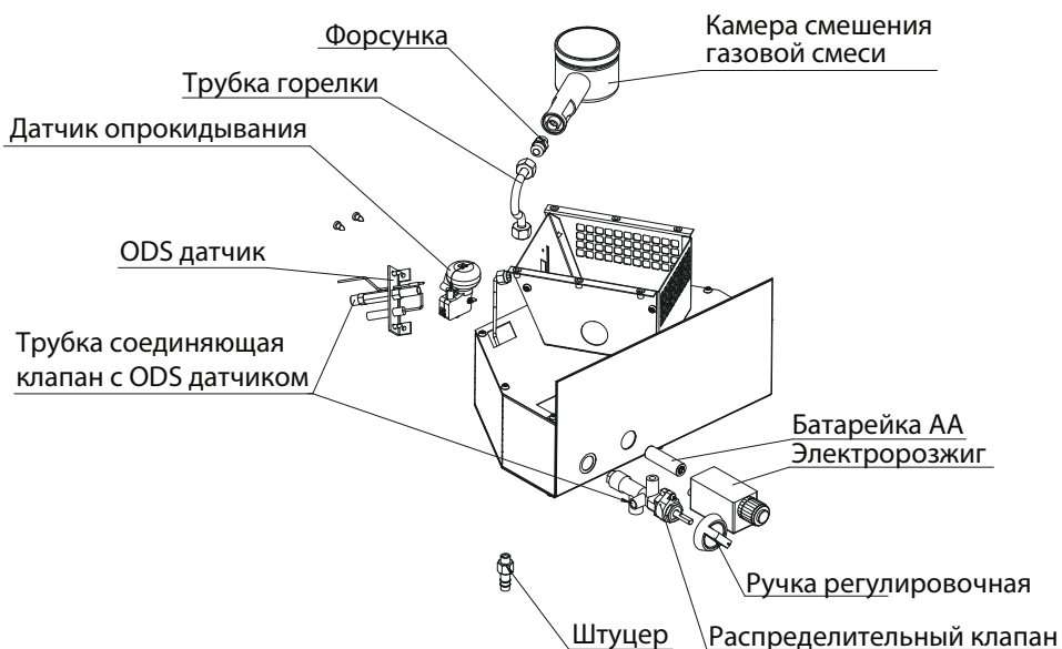
Рис. 3 – Устройство блока управления (приборного отсека)
