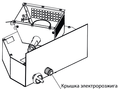
Рис.4 - Замена батареек модели
