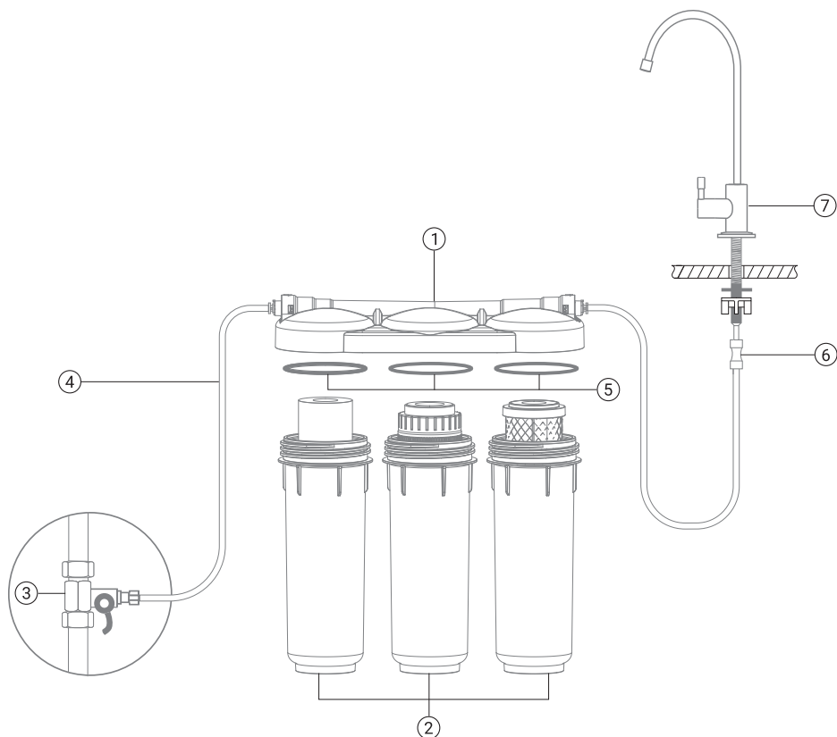
Рис. 1. Схема подключения
