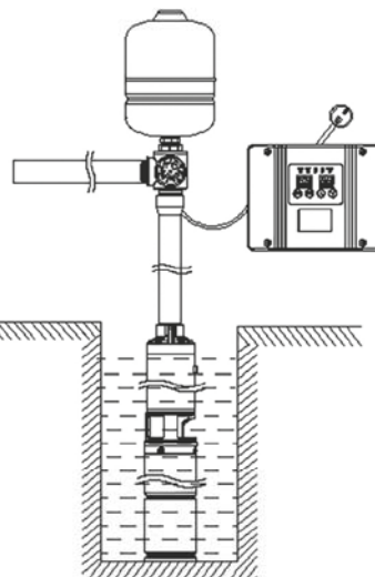
Схема монтажа погружного насоса ↓
