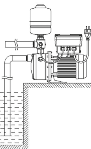
Схема монтажа самовсасывающей насосной станции ↓
