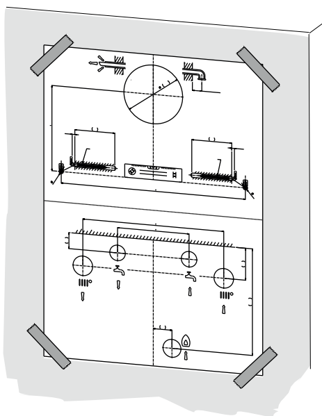
Рис. 31 Монтажный шаблон
