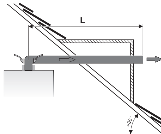
Рис. 3 Горизонтальный отвод дымовых газов B22
