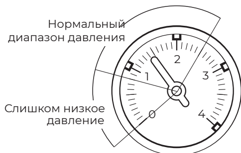
Рис. 12 Показание давления
