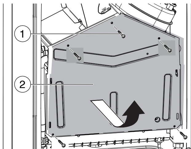
Рис. 26 Открытие горелки
