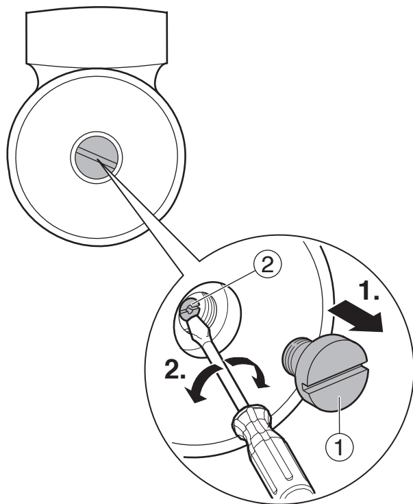
Рис. 30 Разблокировка насоса
