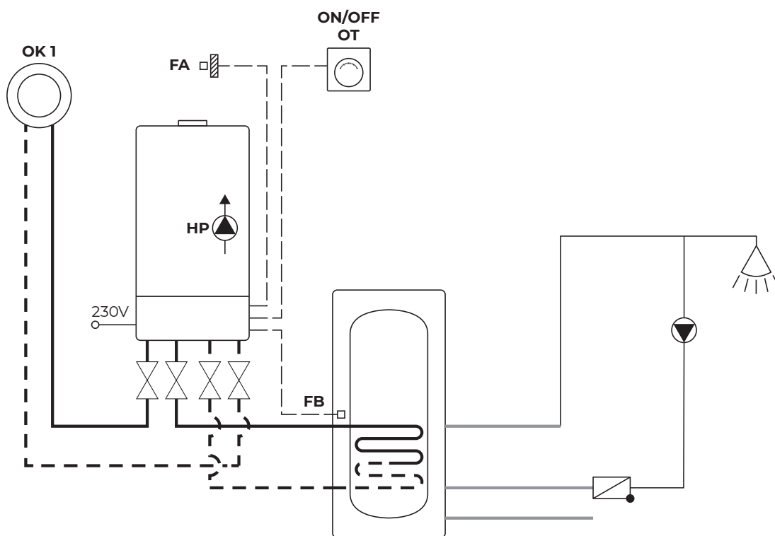
Рис. 37 Схема подключения одноконтурного котла
