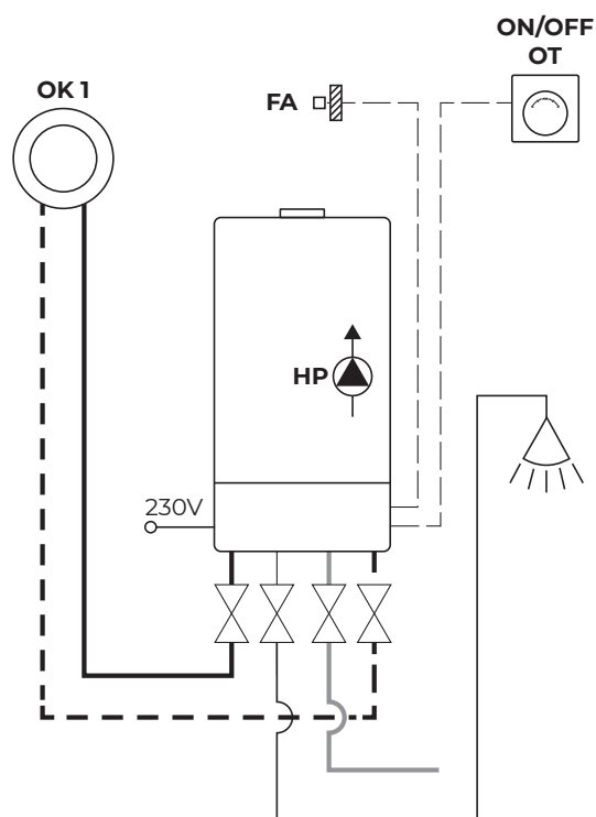
Рис. 36 Схема подключения двухконтурного котла
