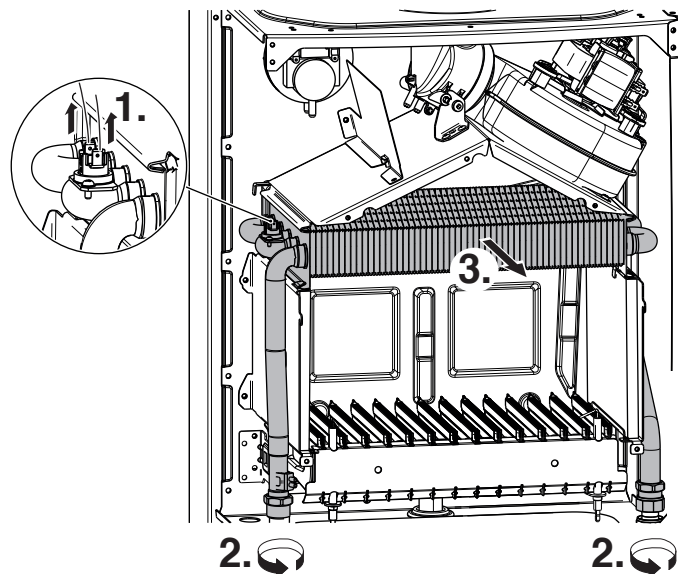
Рис. 28 Чистка теплообменника
