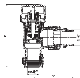
Угловой термостатический клапан
