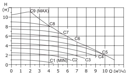
Рис. 14 Кривые режима управления при фиксированной частоте вращения.
