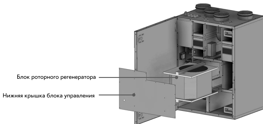
Рис. 28. Обслуживание роторного регенератора
