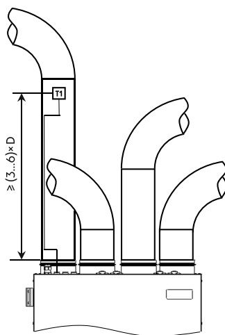
Рис. 10. Установка датчика температуры приточного воздуха
