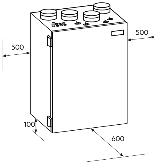
Рис. 6. Сервисное пространство
