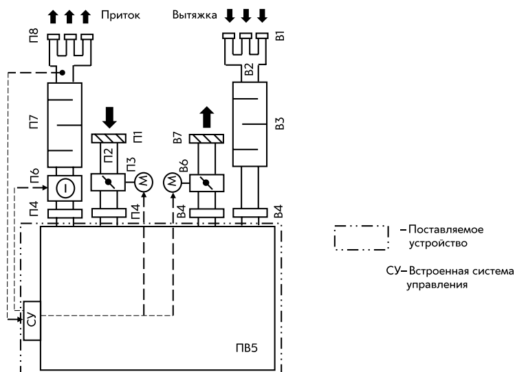
Рис. 3. Рекомендуемая структура и состав системы вентиляции
