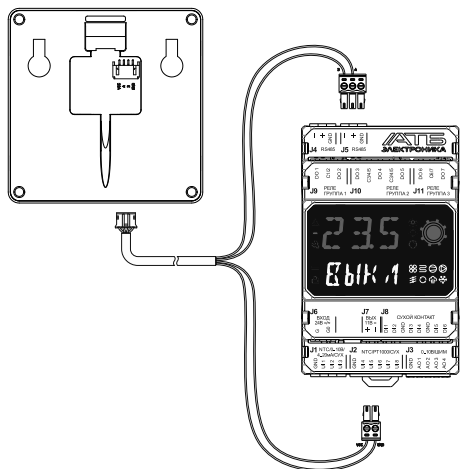
Рис. 13. Подключение к контроллеру
