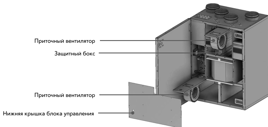
Рис. 29. Обслуживание вентилятора
