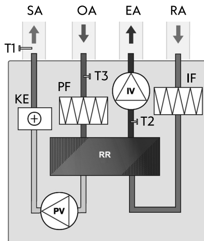
Рис. 2. Принципиальная схема UniMAX-R 300 VE-EC
