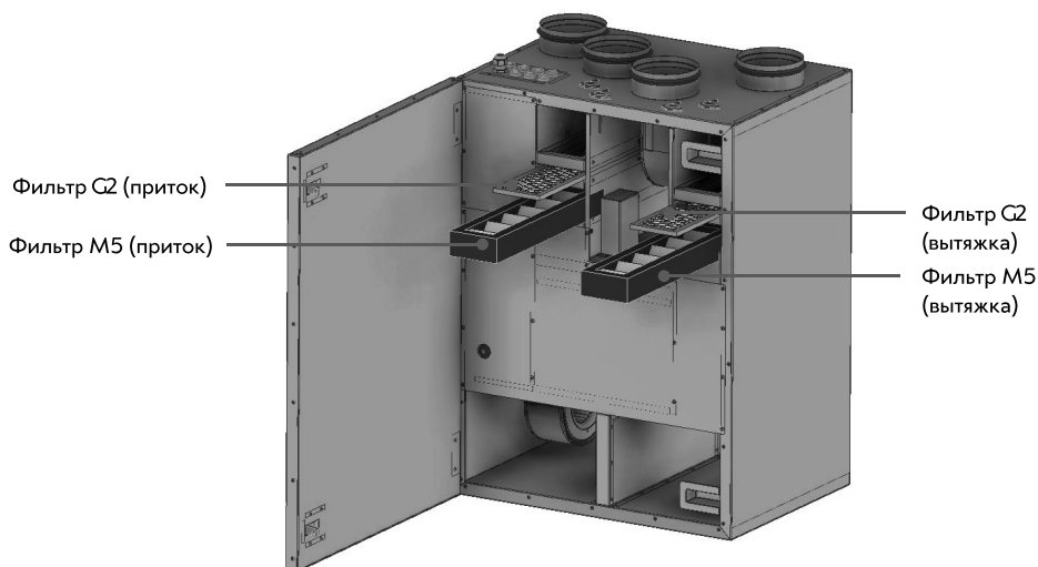
Рис. 27. Замена воздушных фильтров
