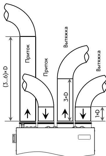
Рис. 7. Рекомендации по длине прямых участков воздуховода
