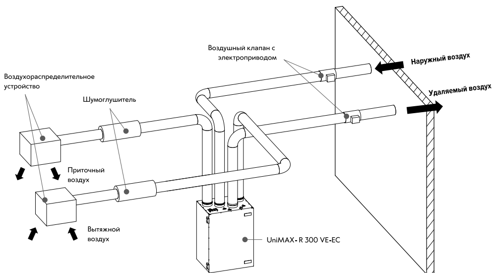
Рис. 9. Монтажная схема
