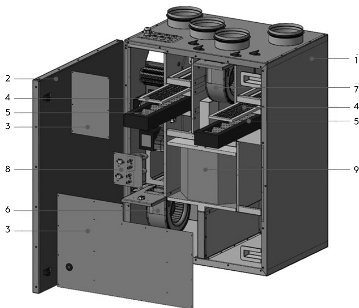
Рис.1. Состав установки UniMAX-R 300 VE-EC
