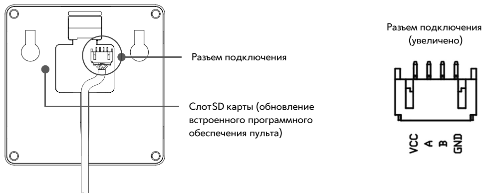
Рис. 12. Подключение к пульта управления
