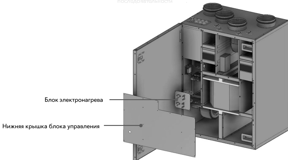
Рис. 30. Обслуживание электронагревателя
