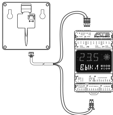
Рис. 6. Подключение к контроллеру
