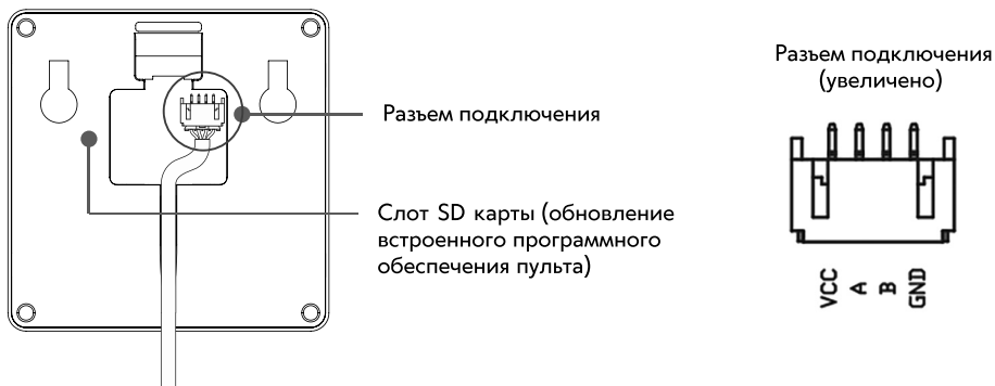
Рис. 5. Подключение к пульту управления
