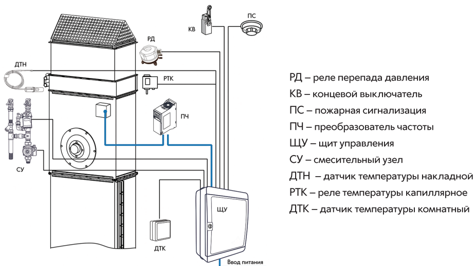
Рис. 30 Функциональная схема. Управление одной завесой с водяным нагревателем.
