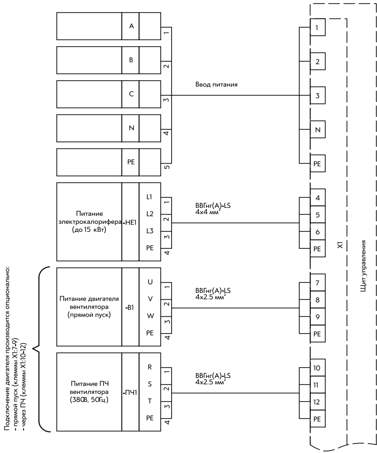
Рис. 36 Схема внешних подключений BM 36-E15-SM340-ZV-ECO. Часть 1.
