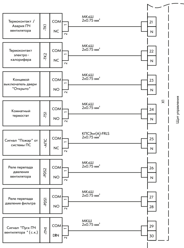
Рис. 41 Схема внешних подключений BM 54-E45-SM375-ZV-ECO. Часть 2.
