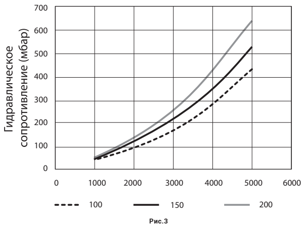
Графики потери напора воды SF100, SF150, SB150, SF200
