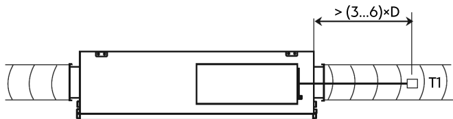
Рис. 18. Установленный датчик температуры приточного воздуха
