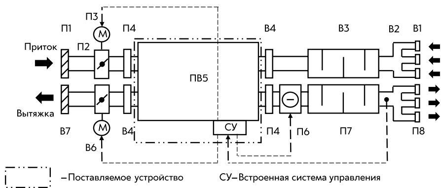
Рис. 6. Рекомендуемая структура и состав системы вентиляции
