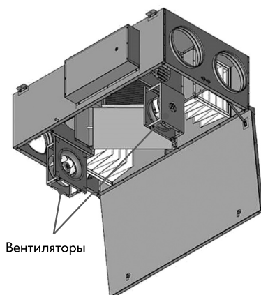
Рис. 38. Обслуживание вентилятора
