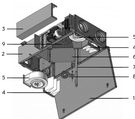
Рис. 1. Состав установки UniMAX-P 450 CE-EC
