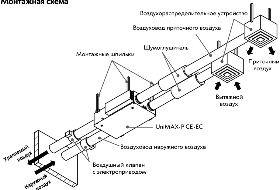
Рис. 16. Монтажная схема
