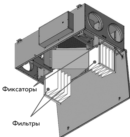
Рис. 35. Замена воздушных фильтров
