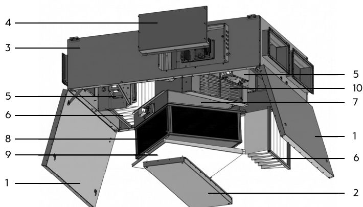
Рис. 3. Состав установок UniMAX-P 1400/2200 CE-EC
