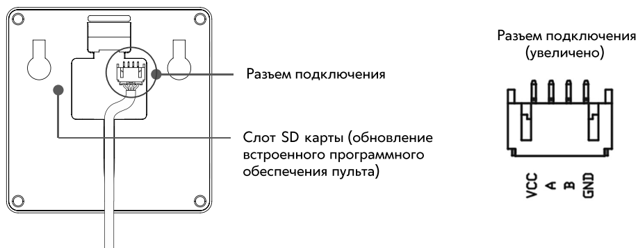
Рис. 19. Подключение к пульту управления
