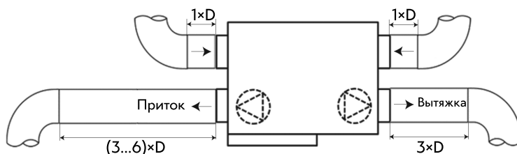
Рис. 12. Рекомендации по длине прямых участков воздуховода
