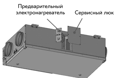
Рис. 40. Обслуживание предварительного электронагревателя
