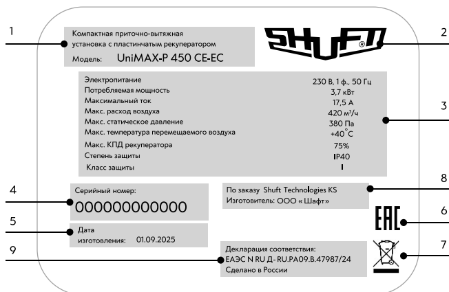
Рис. 7. Пример заводской этикетки
