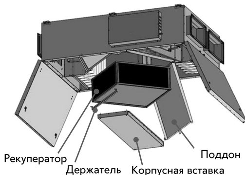
Рис. 37. Обслуживание рекуператора на UniMAX-P 1400/2200 CE-EC
