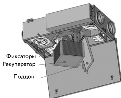
Рис. 36. Обслуживание рекуператора на UniMAX-P 450/850 CE-EC
