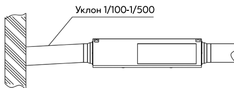
Рис. 14. Уклон наружных воздуховодов
