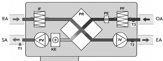
Рис. 4. Принципиальная схема UniMAX-P 450/850 CE-EC
