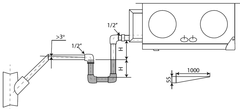
Рис. 15. Дренажная трасса с сифоном
