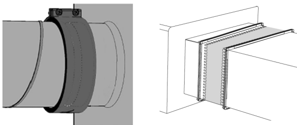
Рис. 13. Подключение воздуховодов
