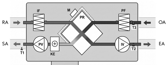
Рис. 5. Принципиальная схема UniMAX-P 1400/2200 CE-EC
