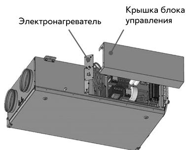
Рис. 39. Обслуживание электронагревателя
