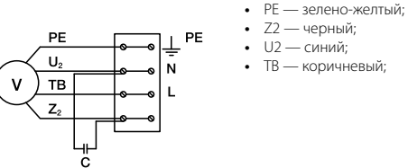
Схема 1 (230 В, 1 ф.)
