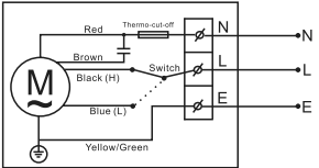
Схема 2 VENTMIX 150, 200
