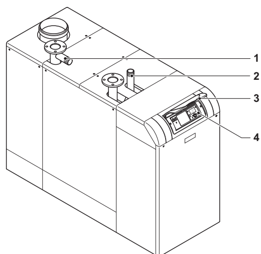
Рис.1 Обзор Power HT-A 1.430 - 1.650
