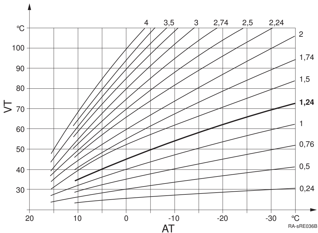
Рис.3 Отопительный график
