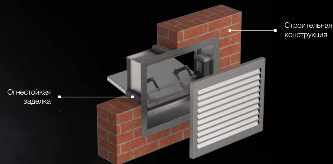
Противопожарные клапаны прямоугольного сечения
