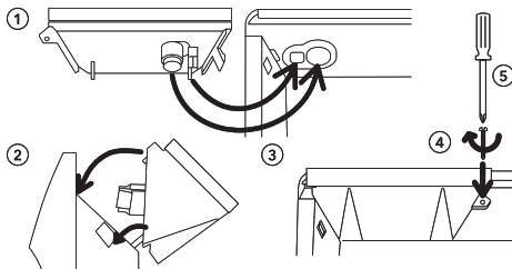
Рис. 3. Схема установки
