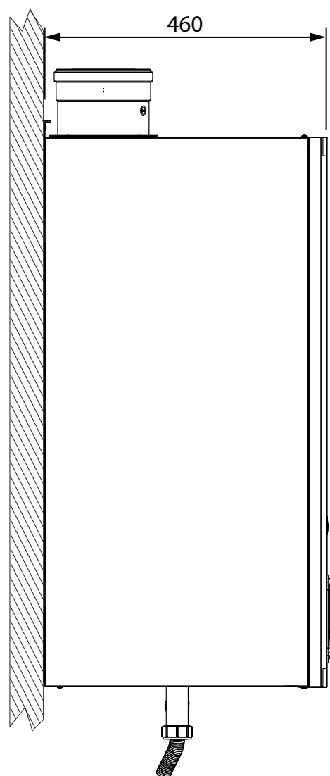
рис. 80- Вид сбоку
