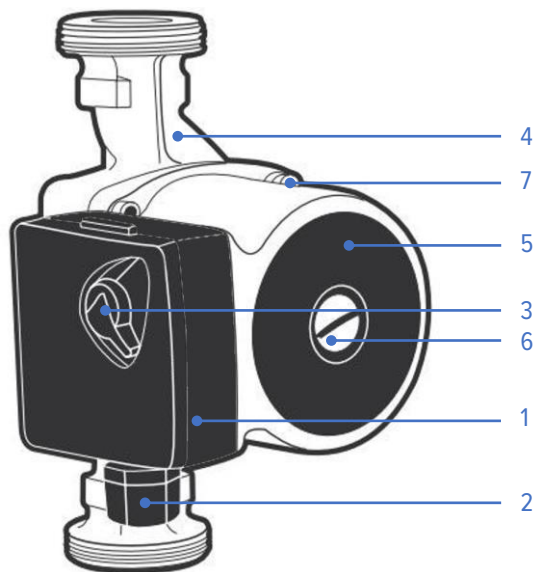
Рис. 10. Основные элементы насоса
