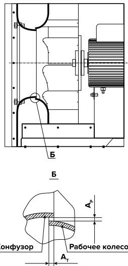
Рис. 3. Зазоры между конфузором и рабочим колесом
