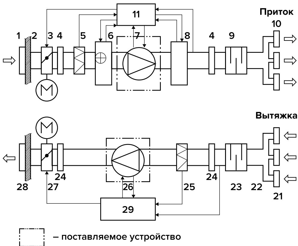
Рис. 1. Структура и состав системы вентиляции.
