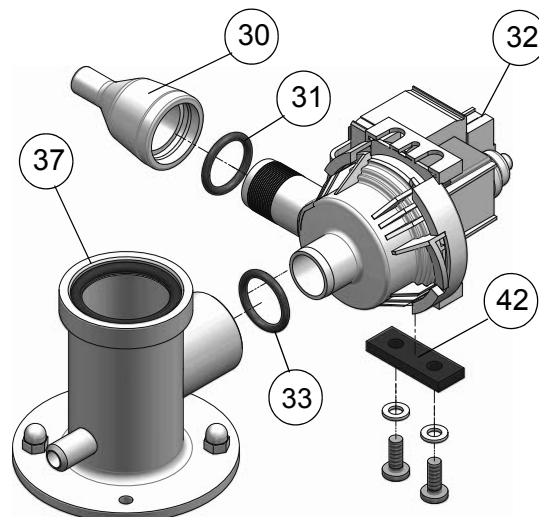
Шламоотводящий насос
