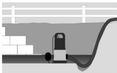
Схема установки электронасоса
