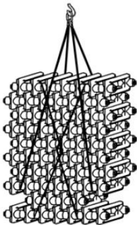
Рис. 2. Пример строповки пакетов.
